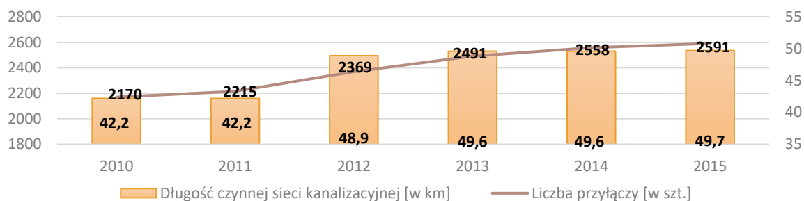
Wykres 10. Długość czynnej sieci kanalizacyjnej i liczba przyłączy w latach 2010-2014
