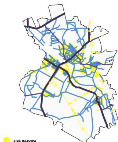
Rysunek 32. Schematyczny rozkład sieci gazowej
